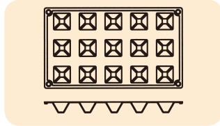
48-03 FRO13 ピラミッド 15ヶ取 単品内寸 高さ (mm) (mm) 36×36(11)×22 791000350
