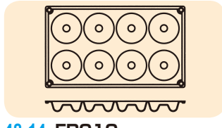
48-14 FRO10 サバラン 8ヶ取 単品内寸 高さ (mm) (mm) 65×21 791000240
