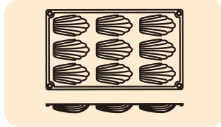
48-02 FRO21 マドレーヌ 9ヶ取 単品内寸 高さ (mm) (mm) 68×45×18 791000310
